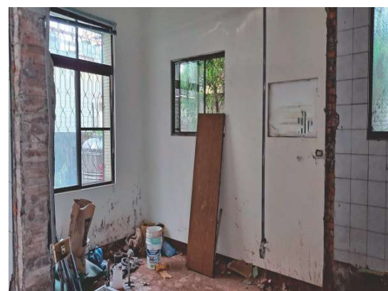
耐震補強施工中照片
