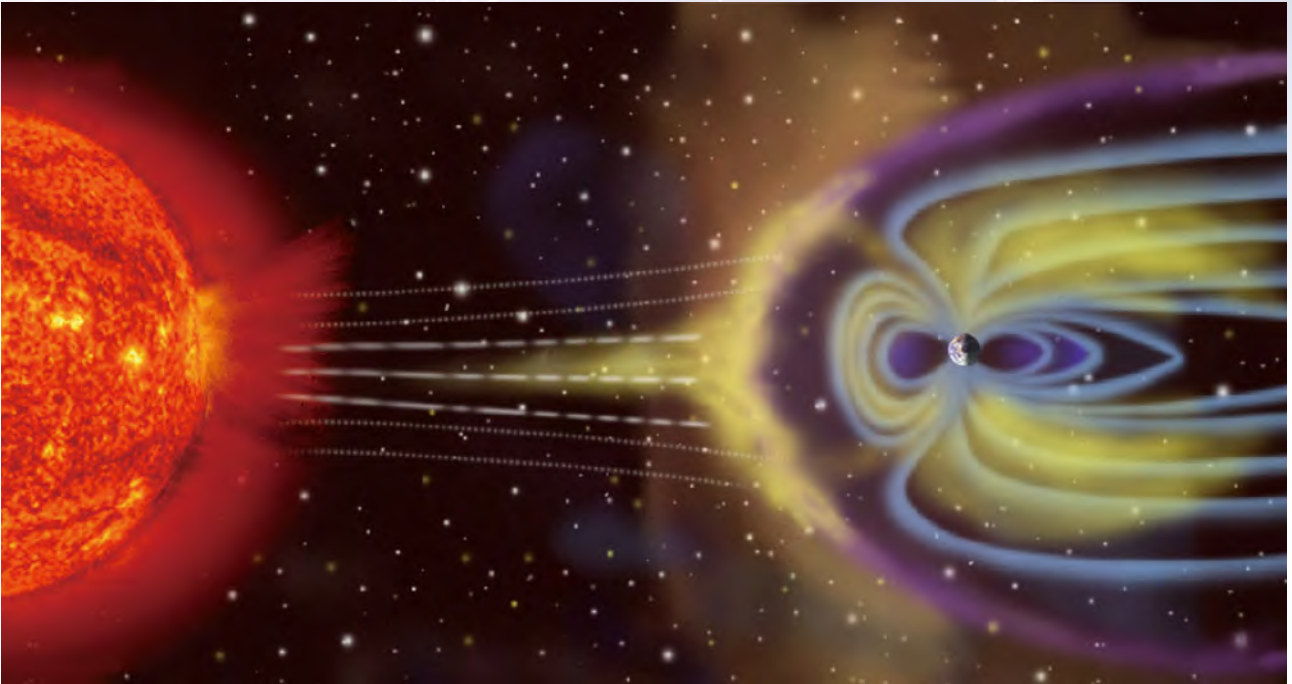
1859 年發生的「卡靈頓事件」是有歷史紀錄以來最強大的太陽風暴，期間產生的磁爆現象會引發短波通訊特性失常、中斷，或使高壓電線產生瞬間超高壓造成電力中斷。圖為太陽風粒子和地球磁層交互作用的示意圖。（Source: NASA, https://commons.wikimedia.org/wiki/File:Magnetosphere_rendition.jpg ）
